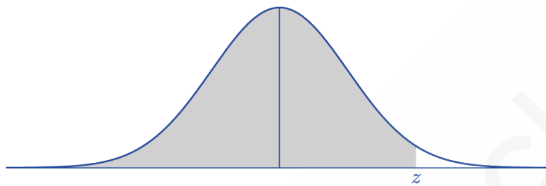
DISTRIBUCIÓN NORMAL
